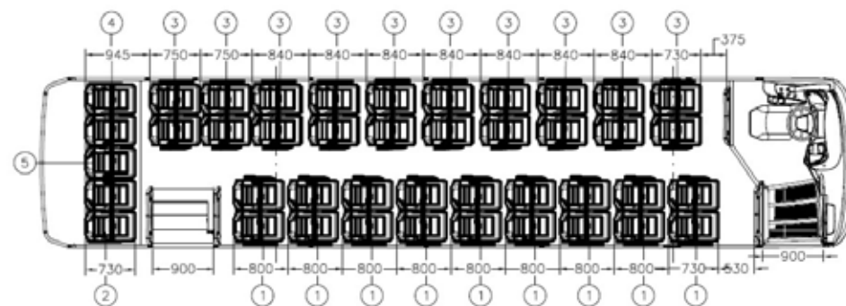
Layout 43 Asientos con dos puertas
