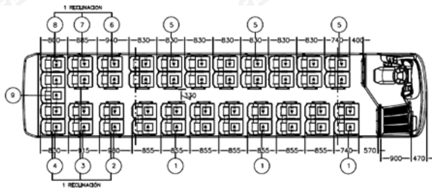
Layout 47 Asientos una puerta
