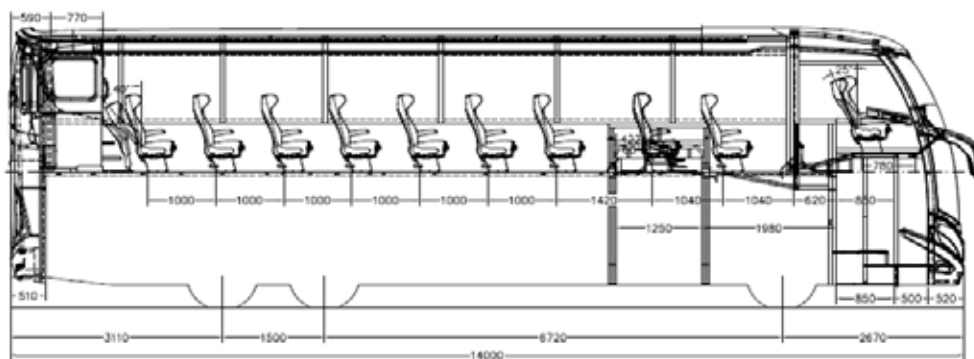
Layout 2 Elevador para silla de ruedas
