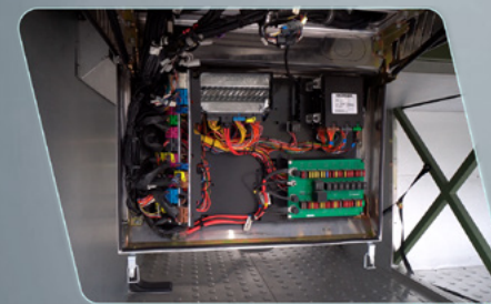
Enrutamiento de chicotes eléctricos, facilitando el mantenimiento y la distribución de los componentes electrónicos.
